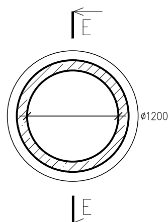
PRZEKRÓJ D-D
